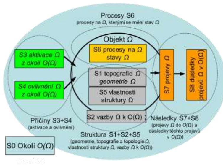
Obr. 13.1: Podmnožiny veličin systému podstatných veličin \Sigma(\Omega)^{34)}
