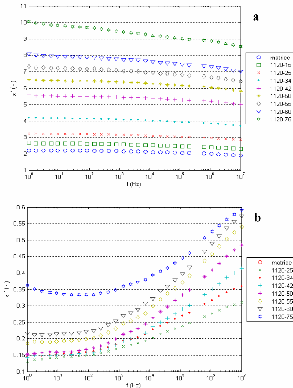
Obr. 5 a) Závislost \epsilon'=F(f) vzorku 1120 při teplotě 297,5 K b) Závislost \epsilon''=F(f) vzorku 1120 při teplotě 297,5 K
