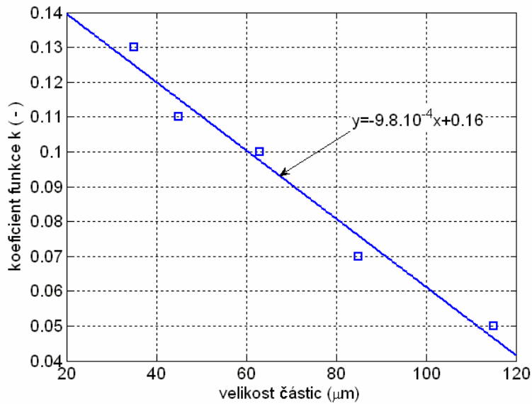
Obr. 11 Závislost koeficientu k z rovnice 4.14 na velikosti dispergovaných částic
