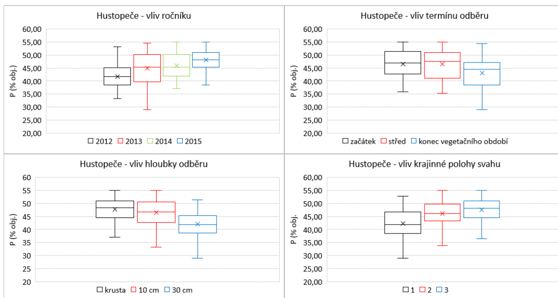
Graf. 7 Průměrné hodnoty pórovitosti v % obj. v lokalitě Hustopeče
