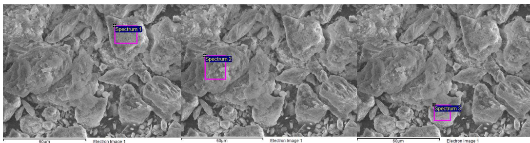
Obr. 2 Spektrální analýza metodou SEM půdní krusty odebrané z plochy F v lokalitě Větrčkovice, transportní zóna (Zdroj: vlastní)
