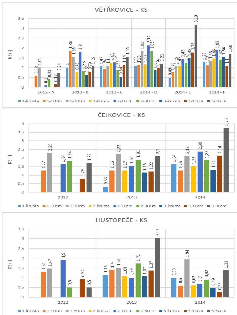
Graf. 8 Koeficient strukturnosti pro experimentální lokality
