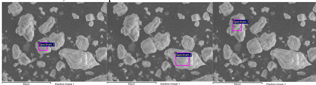
Obr. 5 Spektrální analýza metodou SEM půdní krusty odebrané z plochy C v lokalitě Čejkovice, transportní zóna (Zdroj: vlastní)
