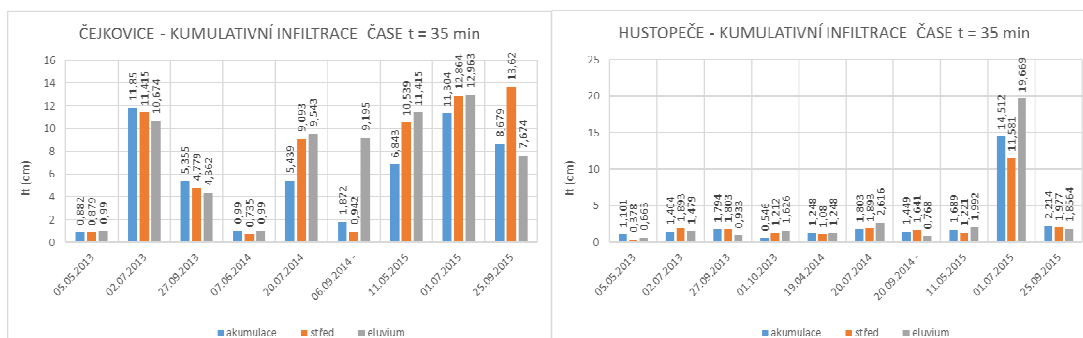
Graf. 10 Kumulativní infiltrace (přepočítaná ze zainfiltrovaného objemu pomocí infiltrační plochy) v čase zasakování t = 35 min
