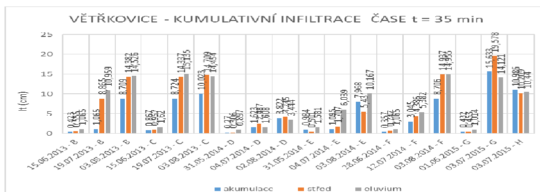
Graf. 9 Kumulativní infiltrace (přepočítaná ze zainfiltrovaného objemu pomocí infiltrační plochy) v čase zasakování t = 35 min
