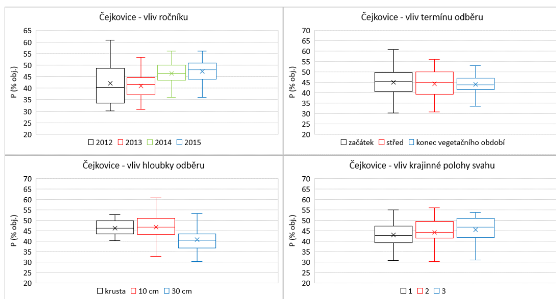
Graf. 6 Průměrné hodnoty pórovitosti v % obj. v lokalitě Čejkovice
