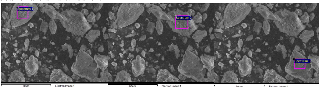
Obr. 3 Spektrální analýza metodou SEM půdní krusty odebrané z plochy F v lokalitě Větrčkovice, eluviální zóna (Zdroj: vlastní)
