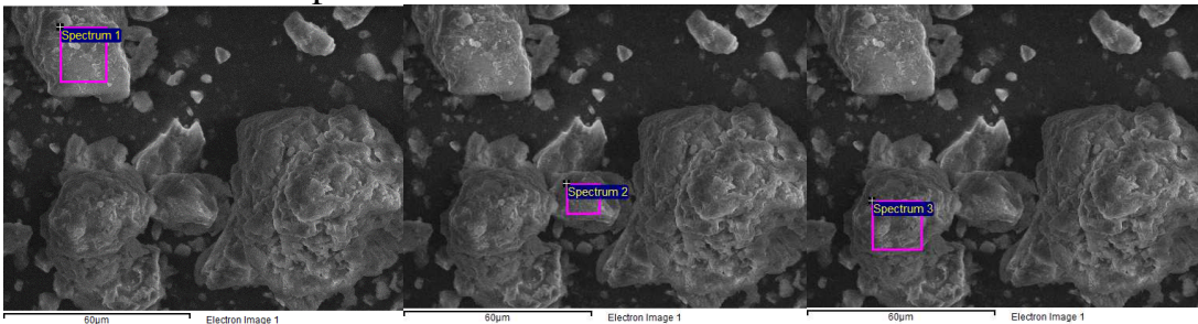
Obr. 4 Spektrální analýza metodou SEM půdní krusty odebrané z plochy C v lokalitě Čejkovice, akumulární zóna (Zdroj: vlastní)
