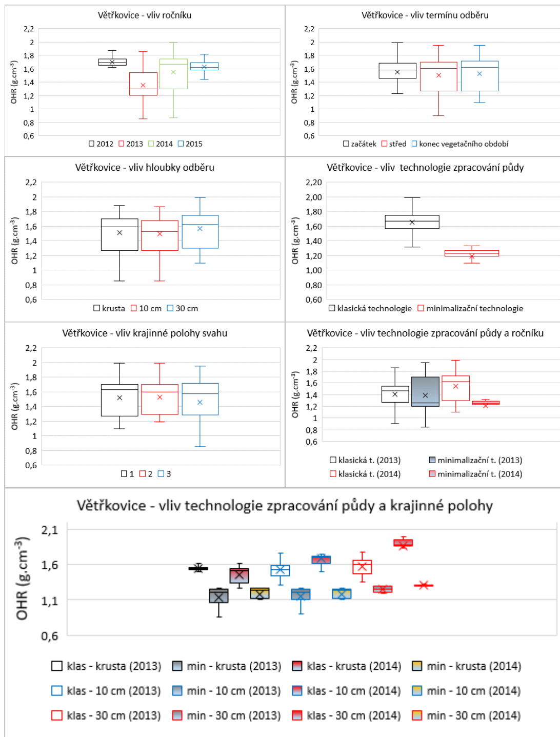
Graf. 1 Průměrné hodnoty obj. hmotnosti redukované v g \cdot cm^{-3} v lokalitě Větrčkovice
