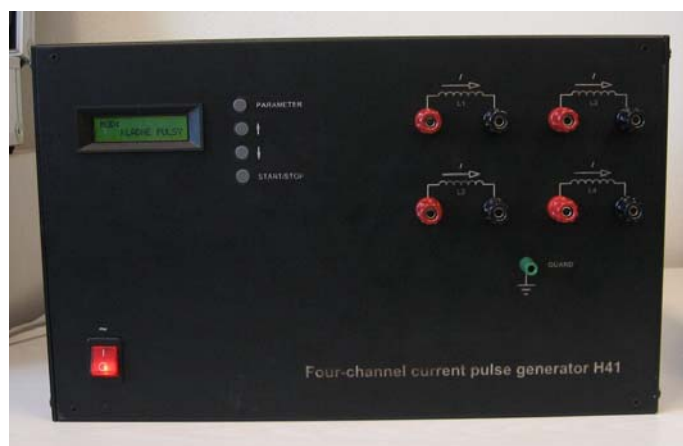
Obr. 6.3 Pohled na čelní panel čtyřkanálového generátoru
