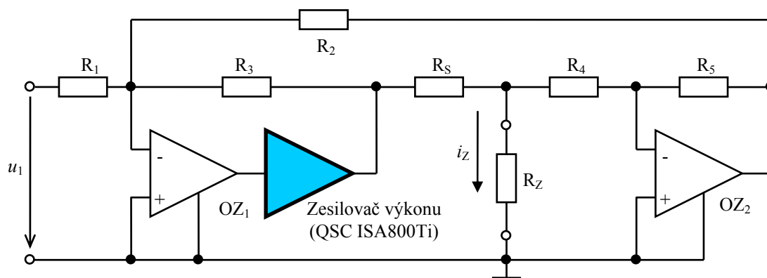
Obr. 6.4 Zdroj proudu řízený napětím s OZ
