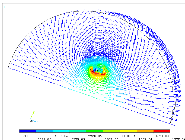
Obr. 5.2 Vektorový potenciál A v soustavě bez jader při proudu I = 55 \text{ A}
