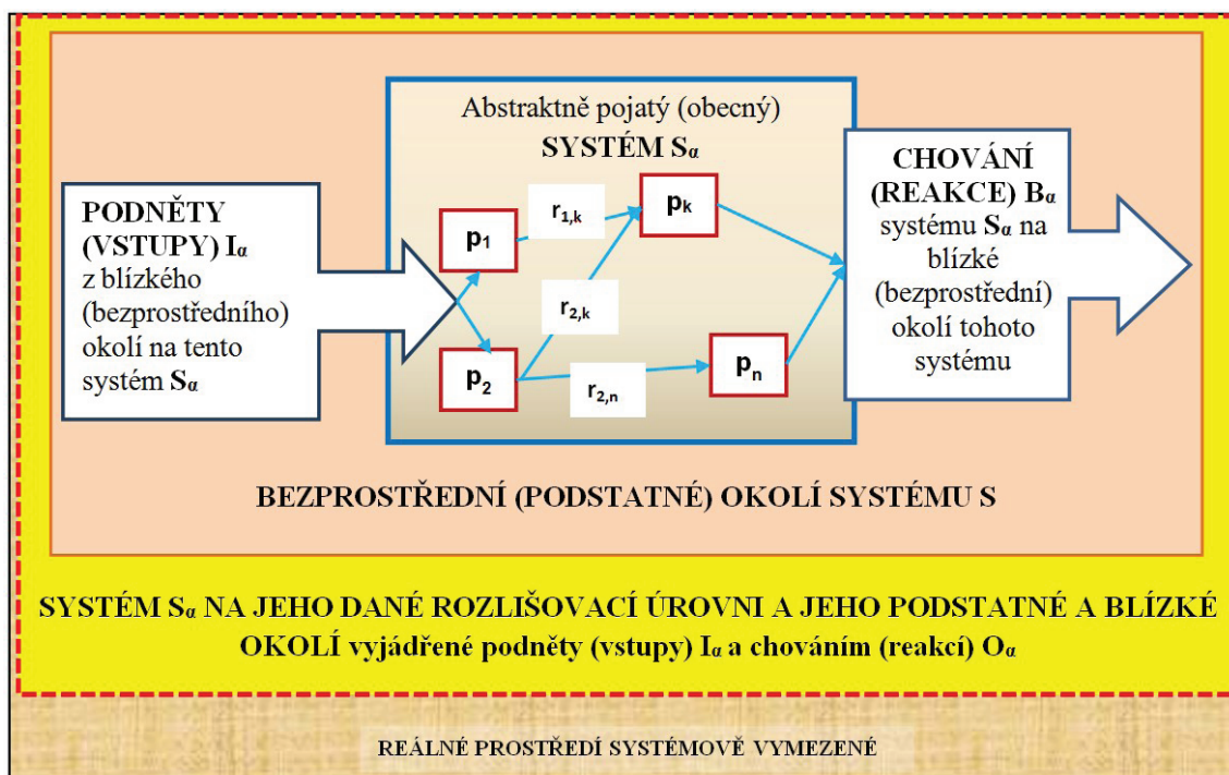
Obrázek 3: Pracovní pojetí abstraktního systému S_\alpha a jeho podstatného okolí
