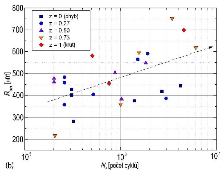
Obr. 7.5 (a) Závislost průměrné hodnoty poloměru rybího oka na vzdálenosti h inkluze pod povrchem. (b) na počtu cyklů do lomu.
