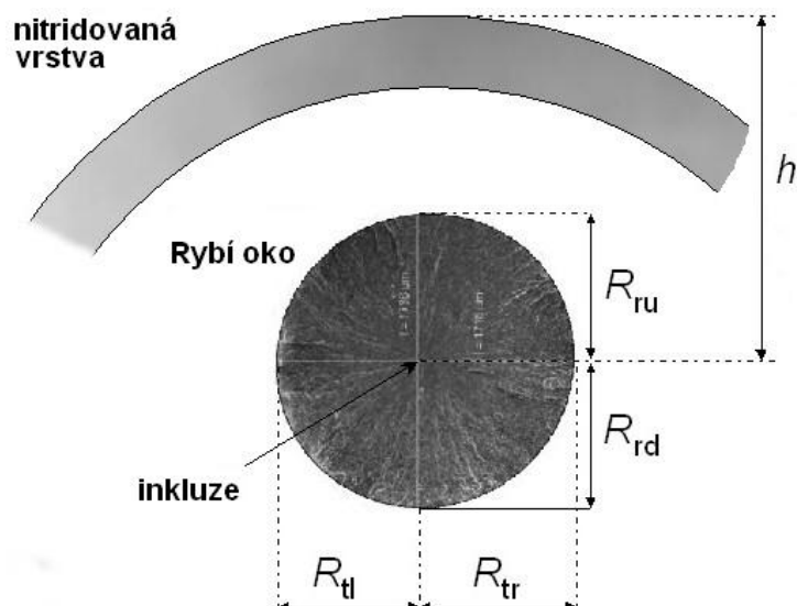
Obr. 7.2 Měřené parametry rybího oka [41].
