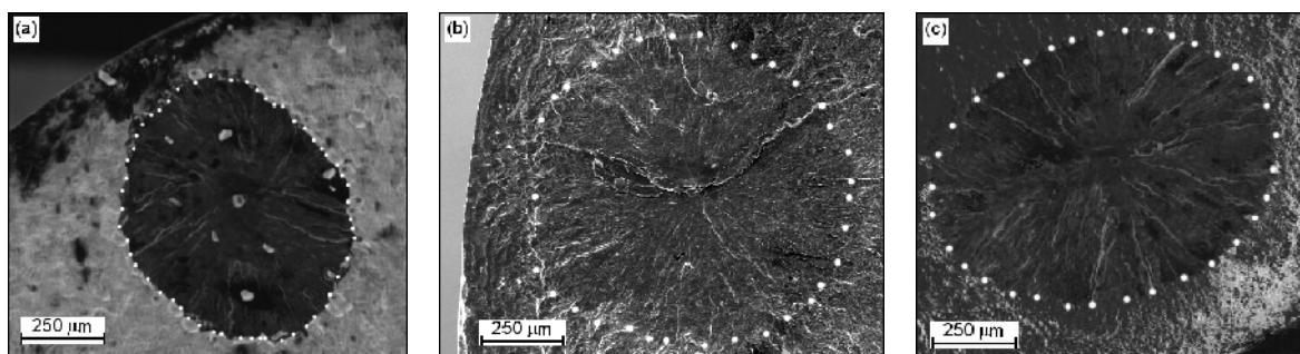
Obr. 7.3 Mikroskopické snímky trhlín typu rybí oko pro různé způsoby zatěžování [41,45]: (a) z = 0 , (b) z = 0,5 , (c) z = 1 .
