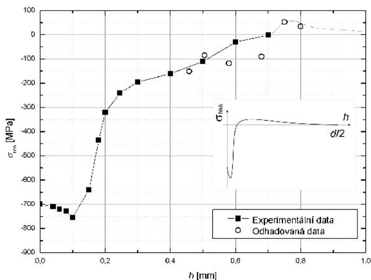
Obr. 7.8 Experimentální profil a teoretický odhad reziduálních napětí v nitridované vrstvě [41]. Na vloženém obrázku je obecné schéma reziduálních napětí podél poloměru vzorku. Experimentální hodnoty vyznačené na tomto obrázku byly získány pomocí RTG měření.
