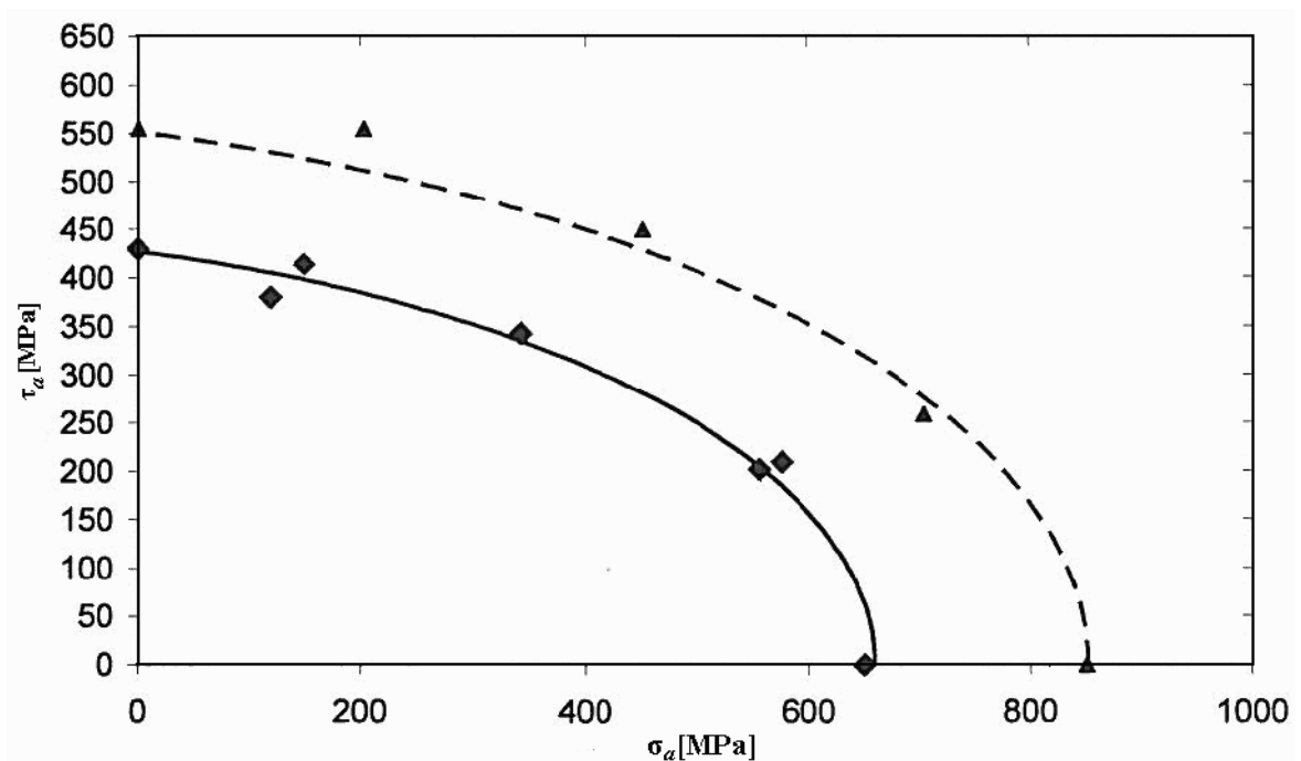
Obr. 3.1 Křivky konstantní životnosti ( N_f = 3 \cdot 10^5 cyklů) pro případ Matakoeva kritéria [12].
