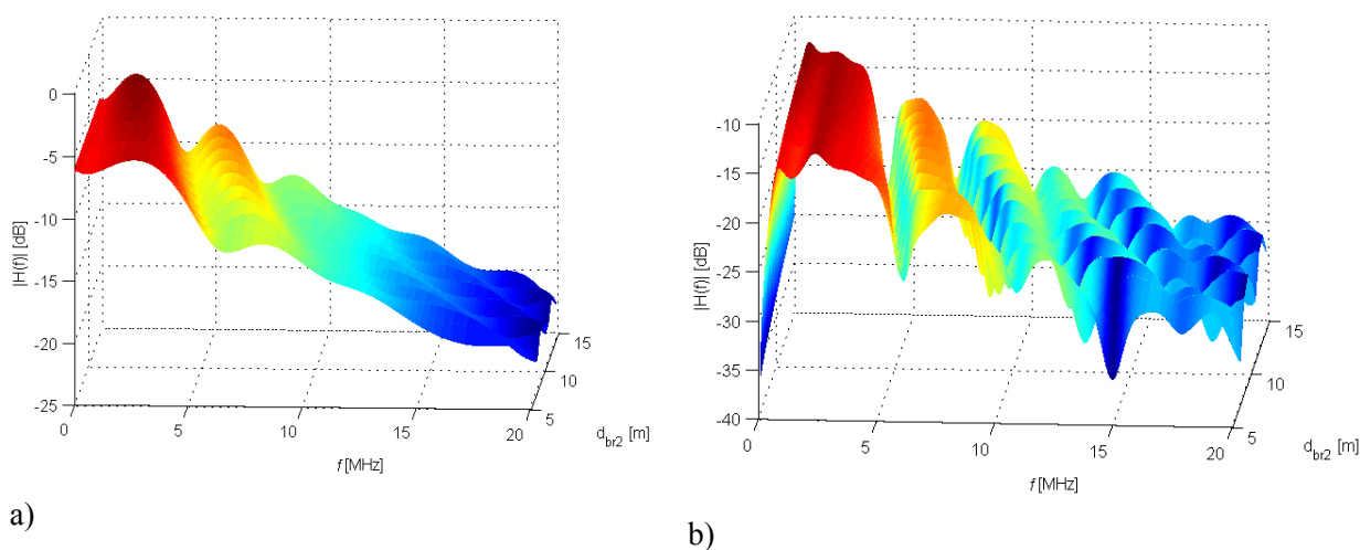
Obr. 4.3: Vliv délky odbočky d_{br2} (C2-C5) na modulovou kmitočtovou charakteristiku vnitřního vedení topologie c) ( a) model vícecestného šíření, b) model kaskádních dvojbranů).
