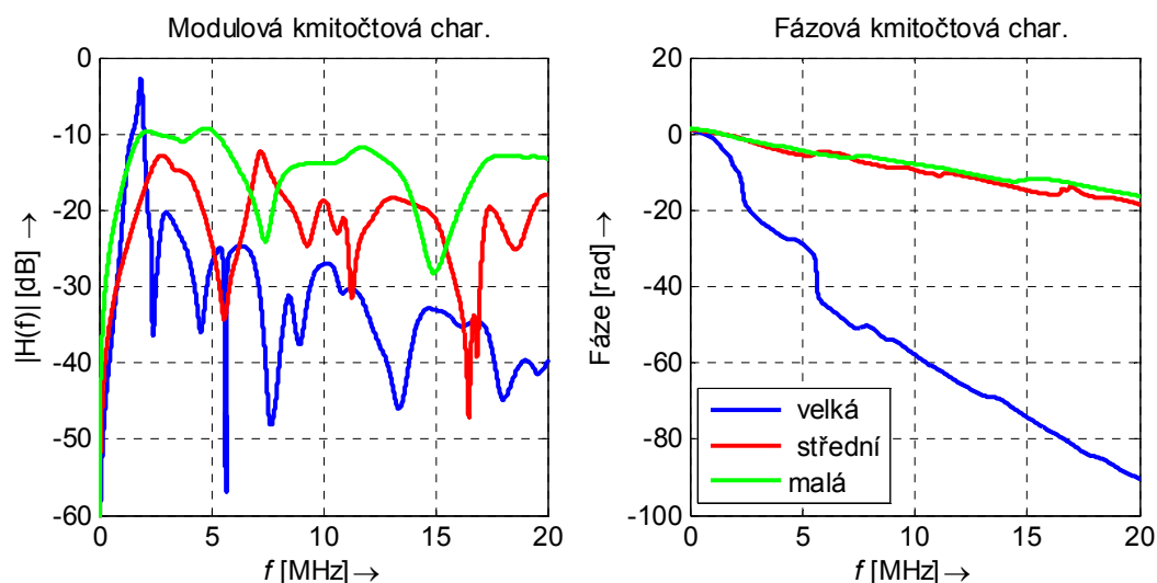
Obr. 4.7: Porovnání přenosových funkcí všech tří topologií s RLC rezonátorem jako impedancí zátěže.
