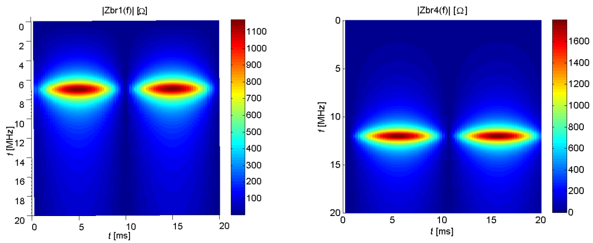
Obr. 4.9: Časově-frekvenční variace impedance zátěže Z_{br1}(Z_{eq1}) a Z_{br4}(Z_{eq3}) .
