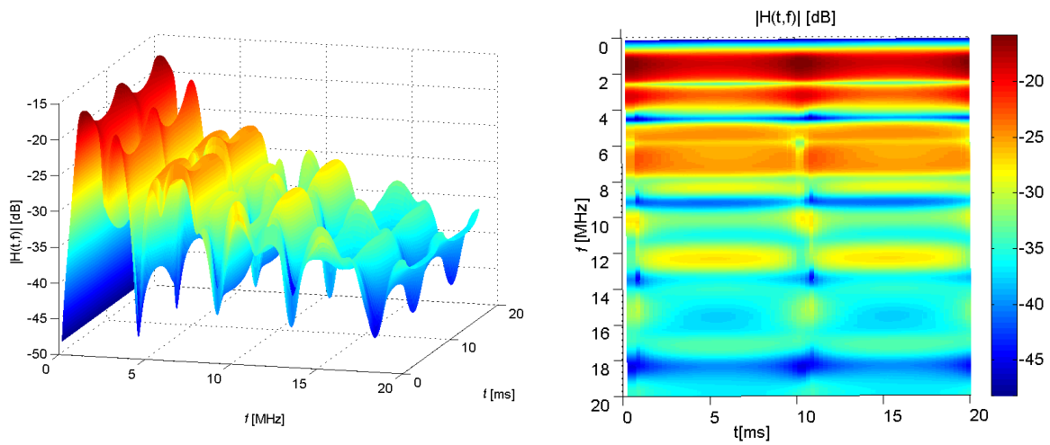
Obr. 4.8: Frekvenční odezva LPTV vedení pro velkou topologii.
