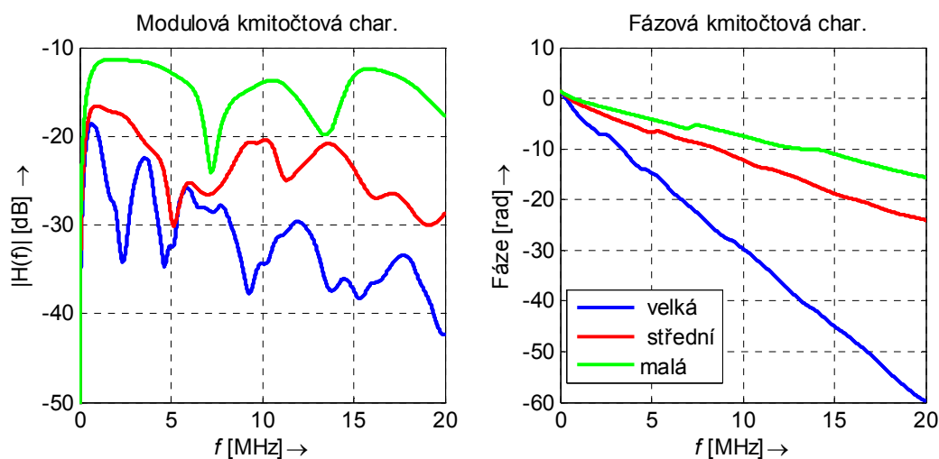
Obr. 4.6: Porovnání přenosových funkcí všech tří topologií s konstantní impedancí zátěže.
