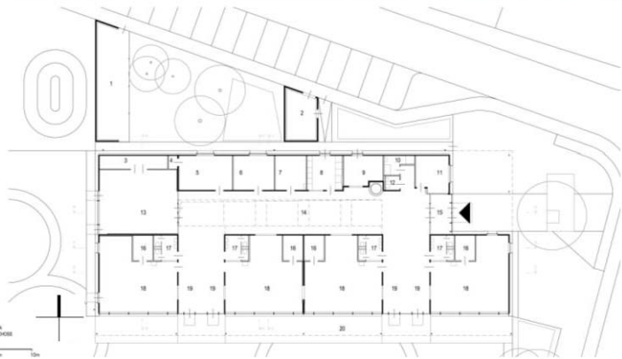
Půdorys. [1]
