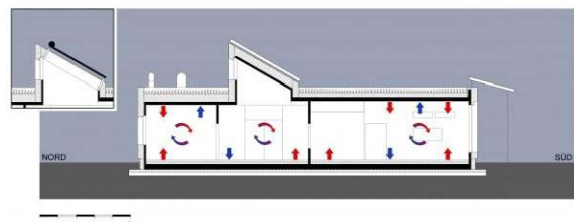
Systém přirozeného větrání – zimní noc. [1]
