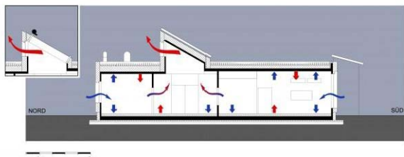
Systém přirozeného větrání – letní noc. [1]
