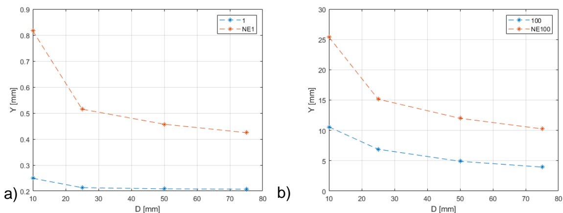
Obr. 7-8 Závislost hloubky průrazu na průměru pro konstantní hmotnost a) 1 b) 100
