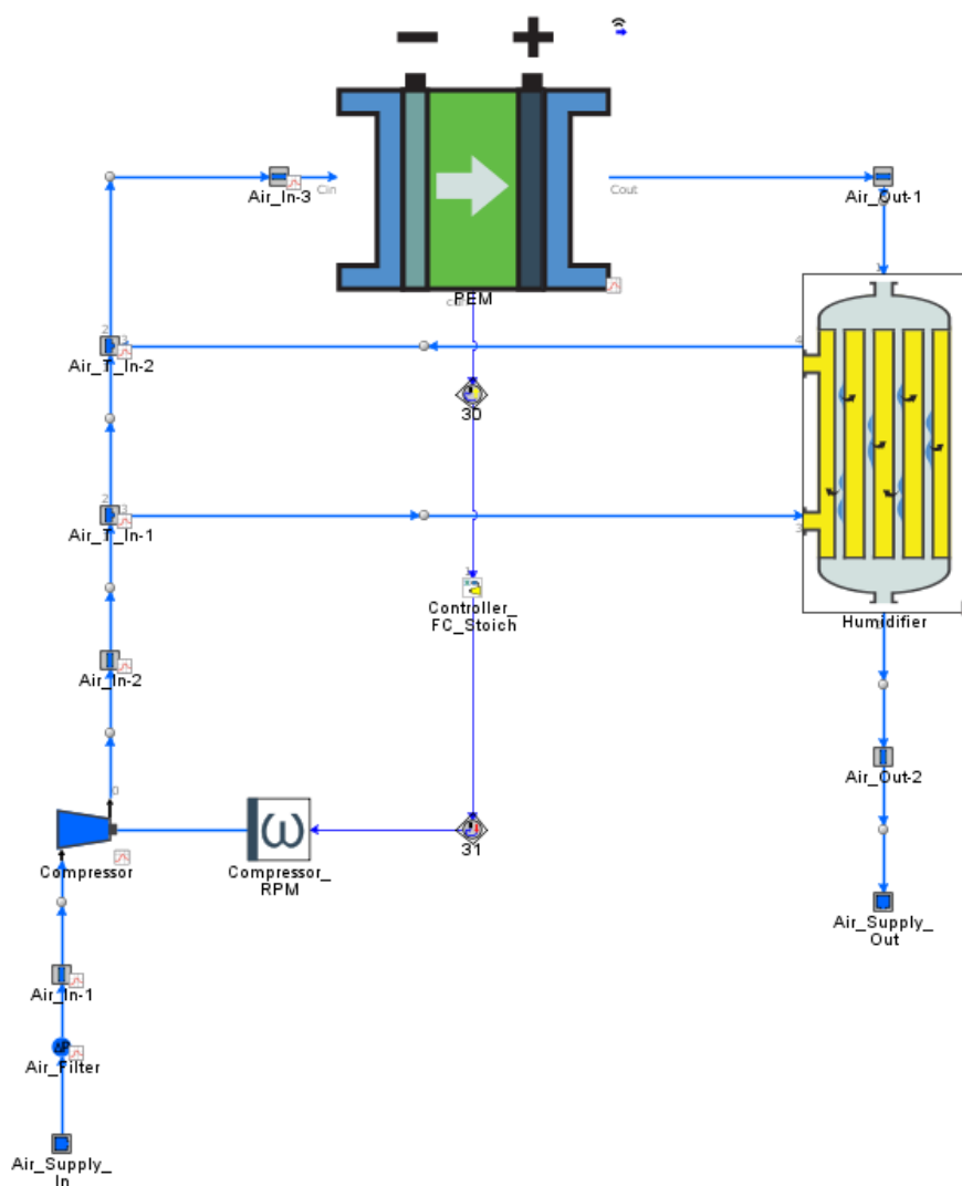
Obr. 22 Subsystém dodávky vzduchu, obsahující vstup do systému, vzduchový filtr, vedení vzduchu, kompresor, zásobník palivových článků, zvlhčovač, řídicí elektroniku a výstup ze systému
