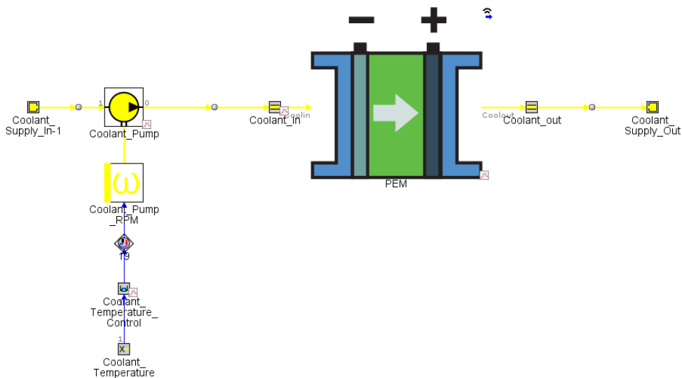
Obr. 25 Subsystém chlazení zásobníku, který obsahuje vstup chladicí kapaliny, chladicí čerpadlo, vedení kapaliny, zásobník palivových článků, řídicí elektroniku a výstup ze subsystému
