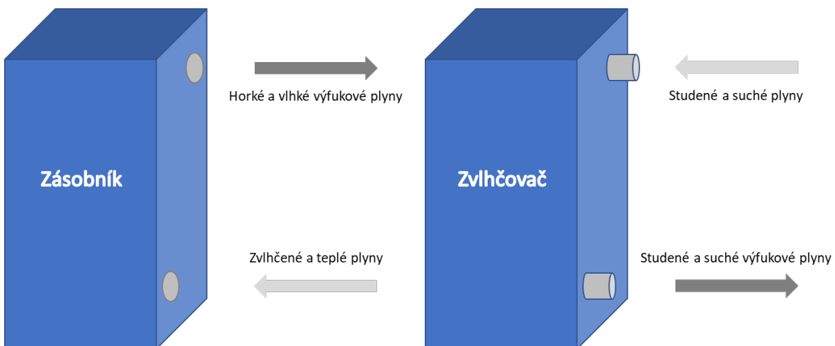
Obr. 9 Základní princip membránového zvlhčovače, který využívá teplo a vodní páru vzniklou při chemické reakci v palivovém článku k ohřevu a zvlhčení suchého vzduchu na vstupu
