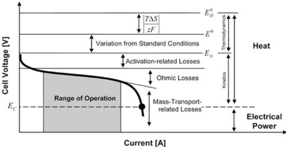
Obr. 5 Provozní napětí palivového článku je dáno napětím naprázdno sníženým o ohmické, aktivací a koncentrační přepětí, která reprezentují ztráty v důsledku fyzikálních a chemických procesů [63]
