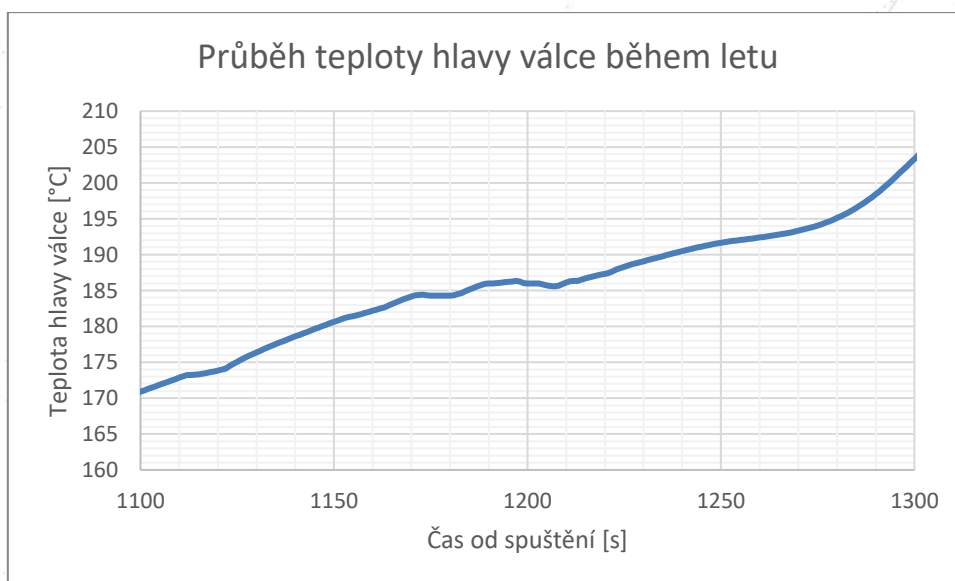
Graf 7 – Vyhlazený průběh teploty
