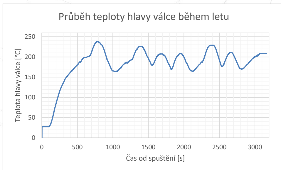
Graf 5 - Průběh teploty hlavy válce během letu
