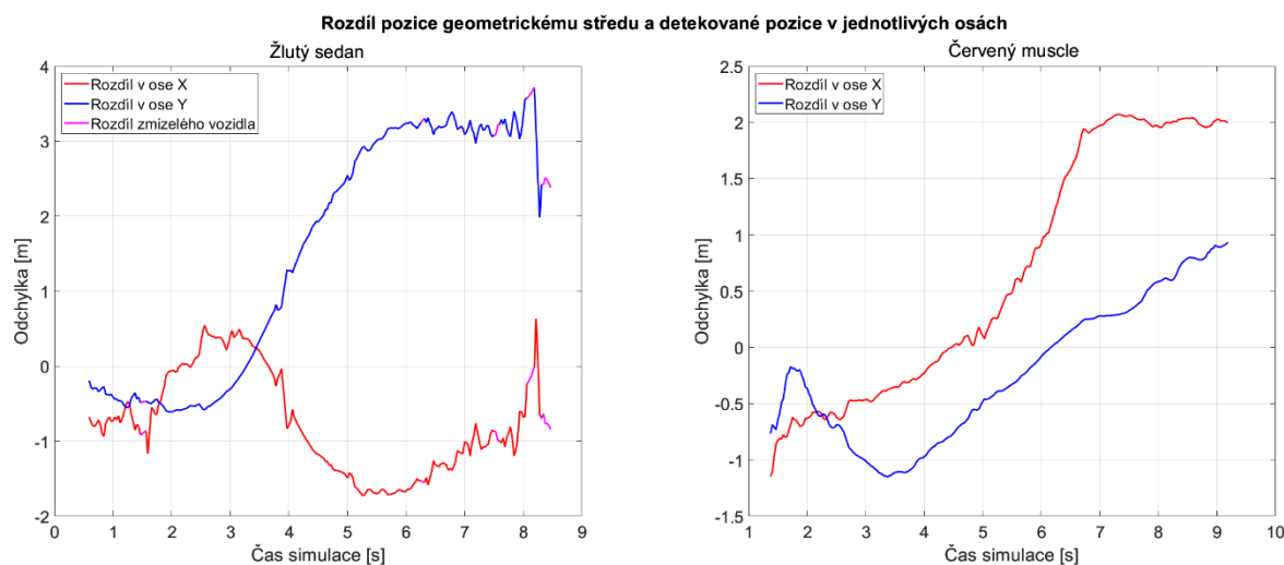
Obr. 54 Odchylka v osách vozidel
