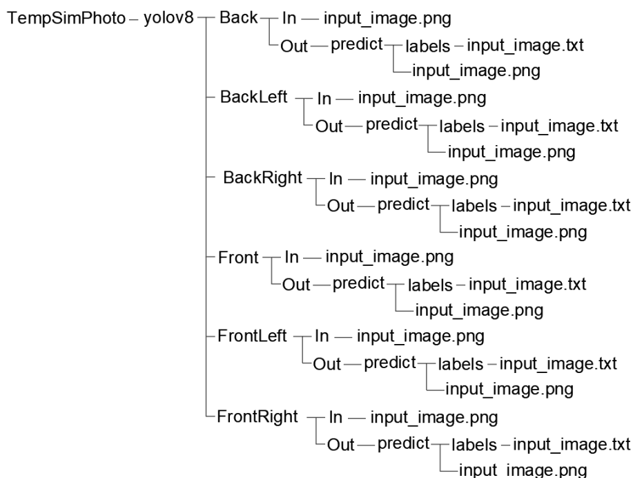
Obr. 39 Struktura adresáře
