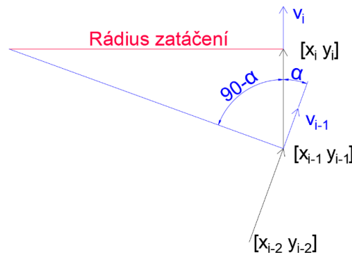
Obr. 47 Znáornění zjednodušeného výpočtu rádiusu zatáčení
