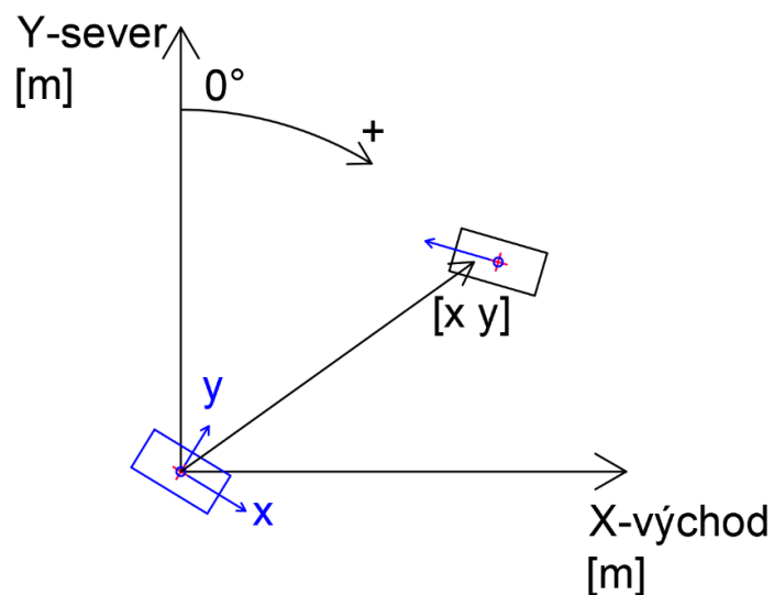
Obr. 18 Lokální relativní kartézská soustava souřadnic
