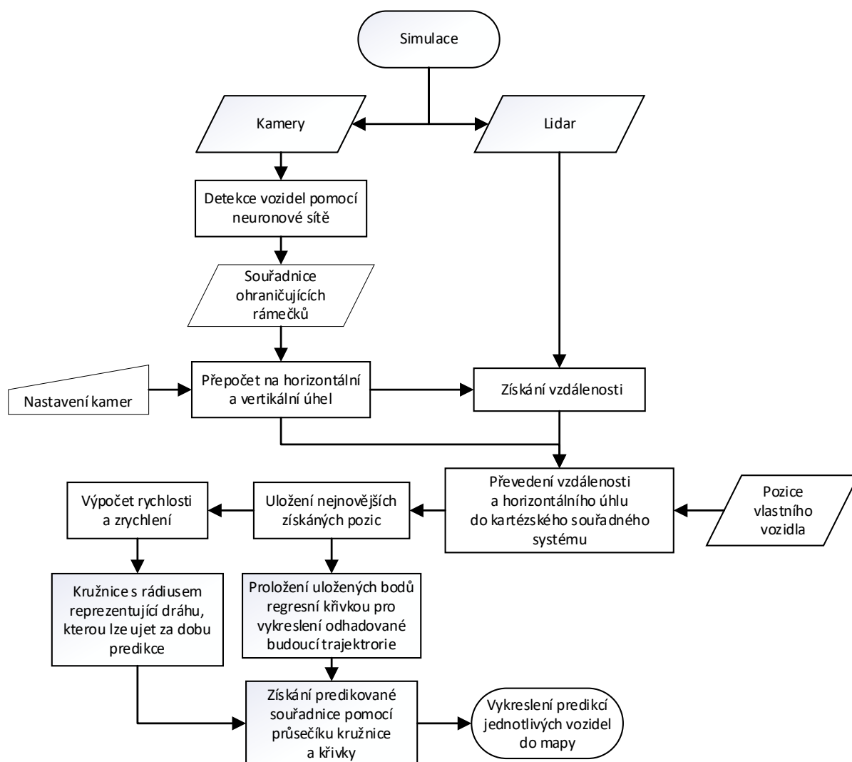
Obr. 33 Logika algoritmu
