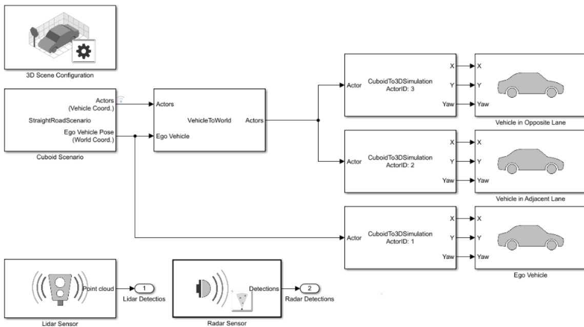
Obr. 27 Rozšířený model [32]
